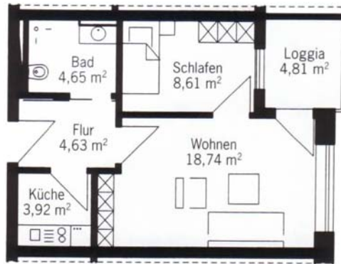
Typ A: 42,96 m 2 Wohnfläche mit Loggia
