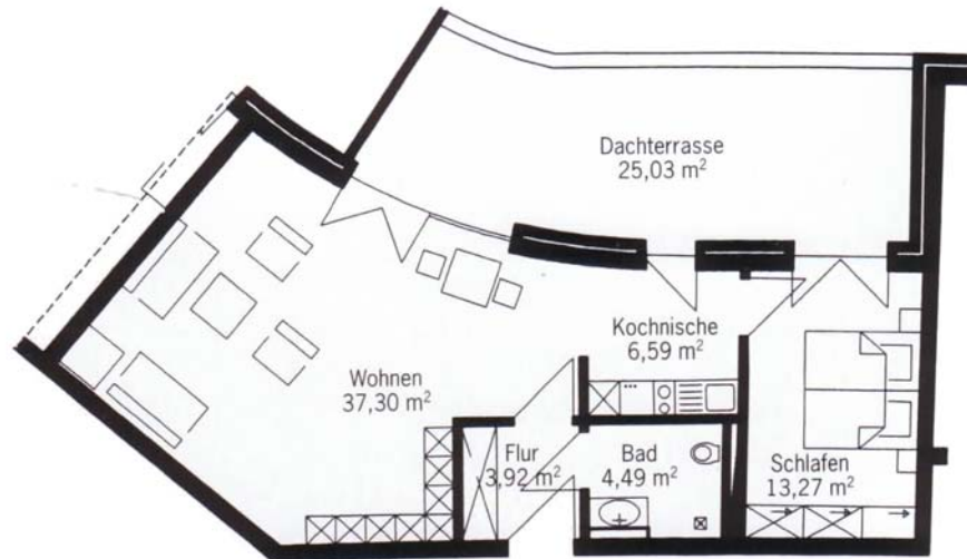
Typ C: 65,57 m 2 Wohnfläche mit Dachterrasse
